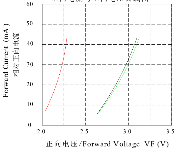
Forward Current vs. Forward Voltage (Ta=25°C) 正向电流与正向电压曲线图
